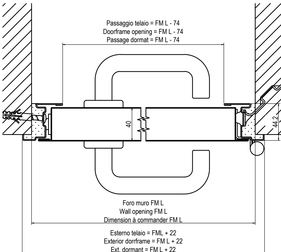
Sezione orizzontale Horizontal cross section Coupe horizontale
